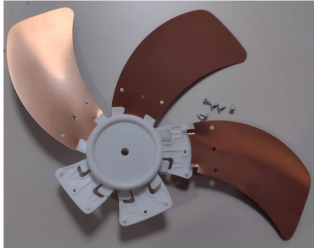
2) Inserte el aspa en la ranura
