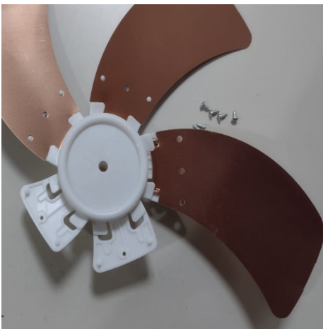
3) Calce el aspa en las trabas
